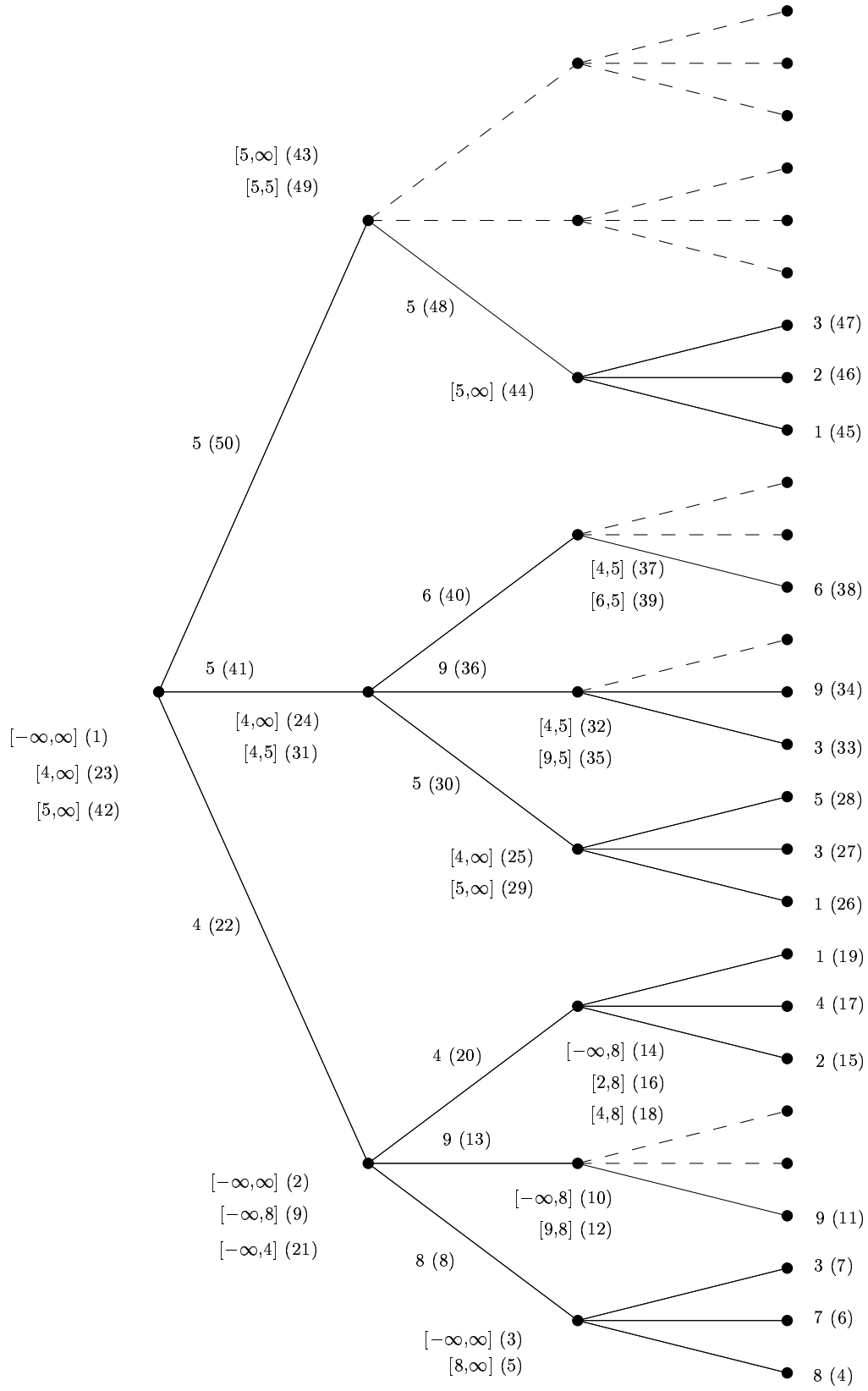
FIG. 1 – Exemple de recherche par l'alpha-bêta
